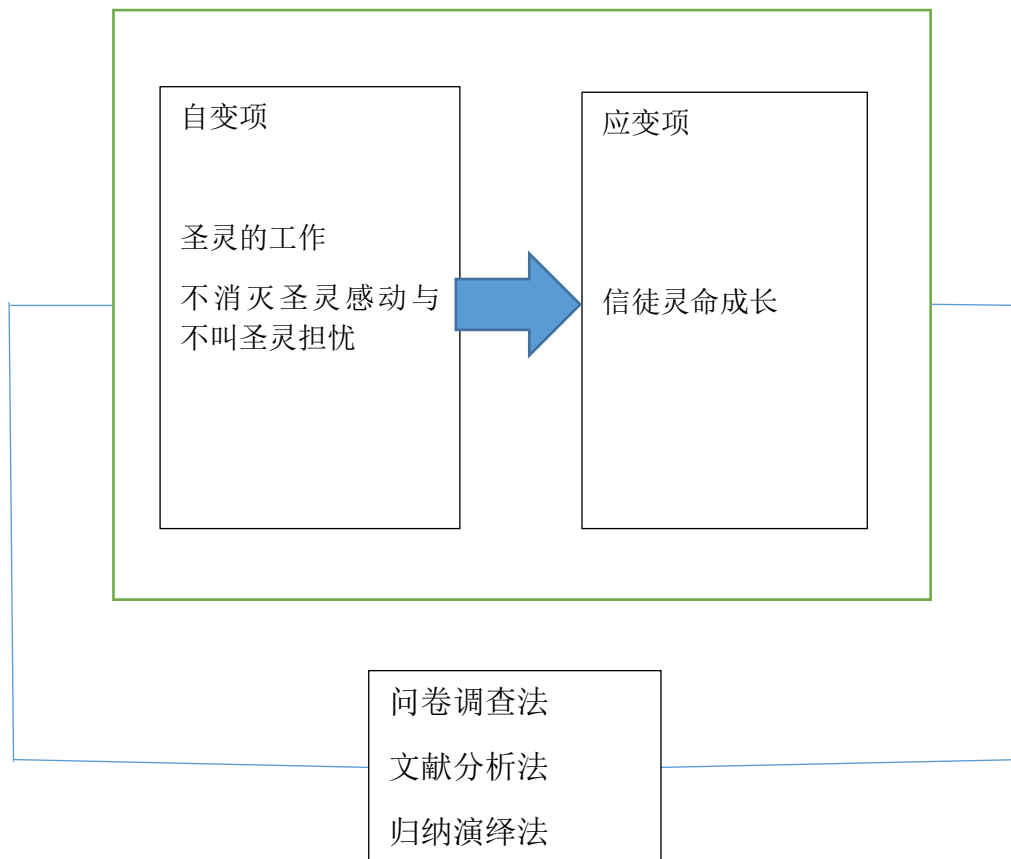
图 1-2-1: 研究架构图
